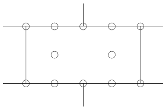
Figure 1a : Plans de chevillage – panneaux de dimensions 1000 × 500 mm
